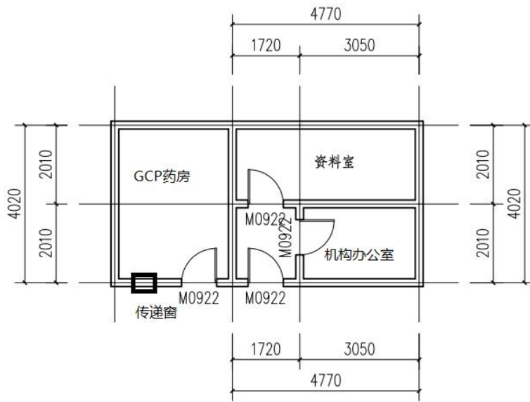
5号楼2楼GCP平面图 1:100
