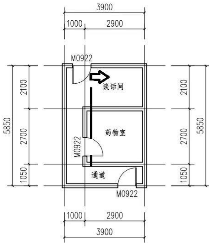
1号楼3楼心血管一区 1:100
