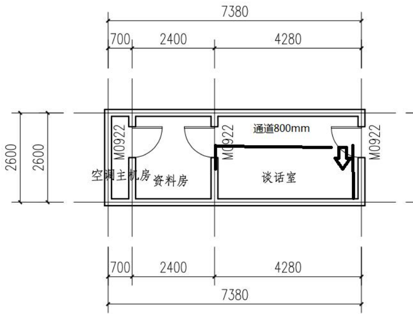
5号楼1楼公共区域 1:100
