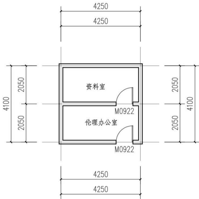
5号楼2楼CCP 1:100
